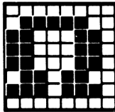
191 &HBF &X10111111
