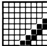
194 &HC2 &X11000010
