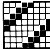
200 &HC8 &X11001000
