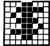
36 &H24 &X00100100
