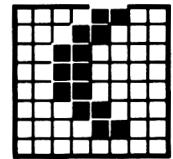
40 &H28 &X00101000
