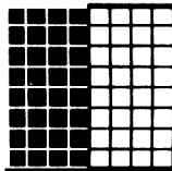
133 &H85 &X10000101
