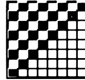
220 &HDC &X11011100
