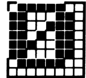
48 &H30 &X00110000
