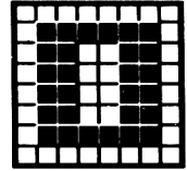
232 &HE8 &X11101000
