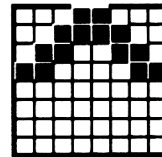
196 &HC4 &X11000100
