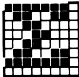
190 &HBE &X10111110
