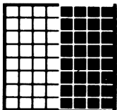
138 &H8A &X10001010
