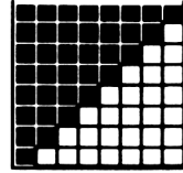
212 &HD4 &X11010100
