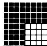
135 &H87 &X10000111
