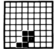
44 &H2C &X00101100
