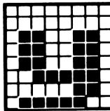
121 &H79 &X01111001
