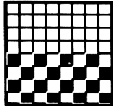
218 &HDA &X11011010
