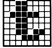
116 &H74 &X01110100
