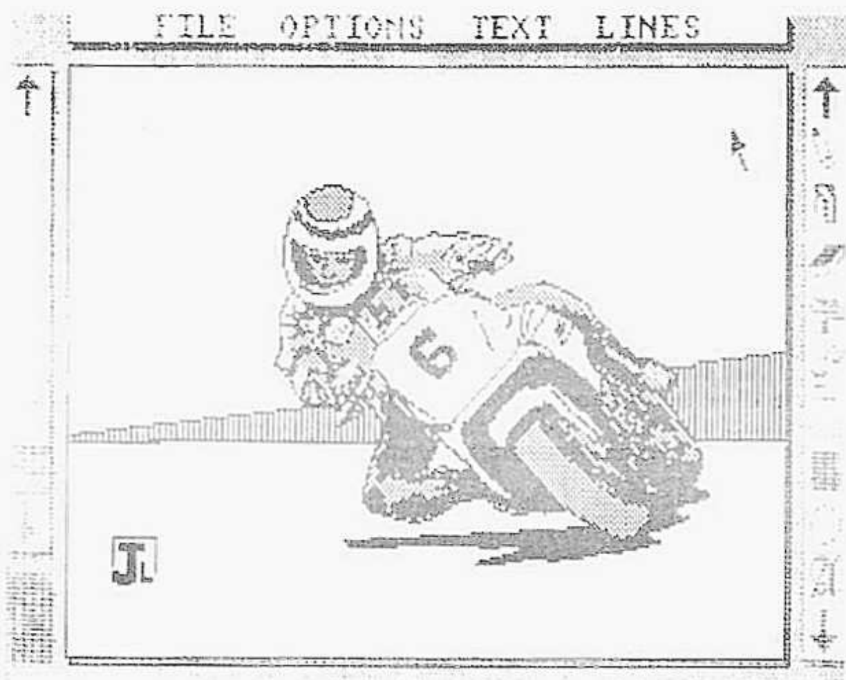
Figure 3 - L'écran "ART"
