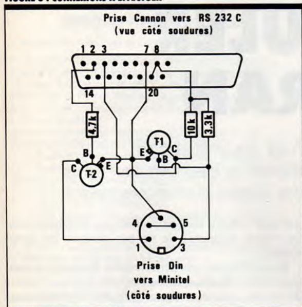
FIGURE 3 : CONNEXIONS A EFFECTUER
