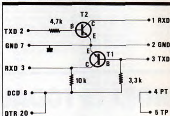
FIGURE 1 : LE BRANCHEMENT THÉORIQUE
